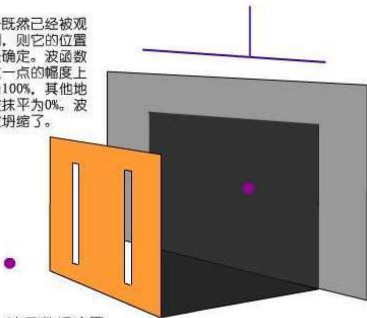
图5：波函数坍缩了
